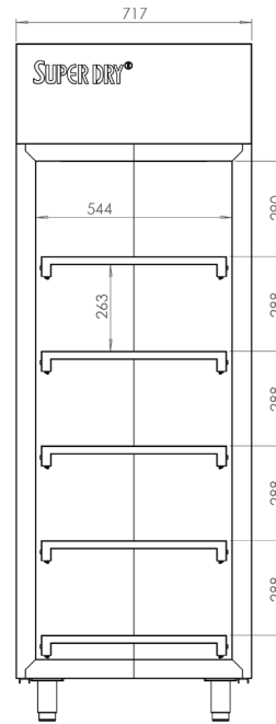
Frontansicht
