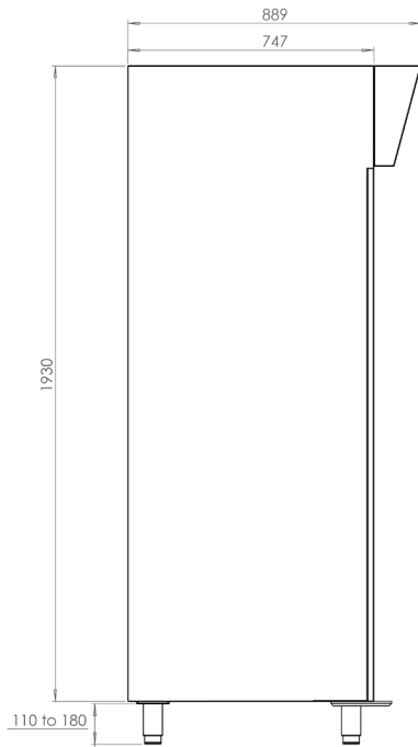
Seitenansicht
