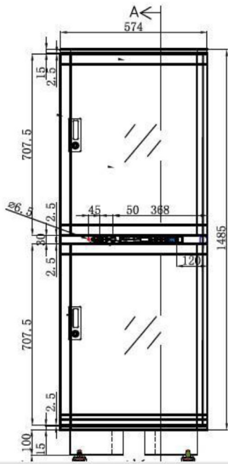
Frontansicht
