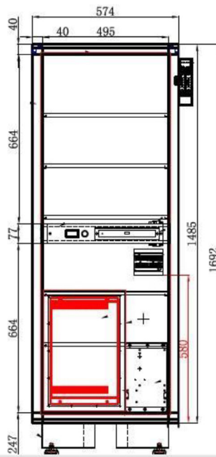
Rückansicht
