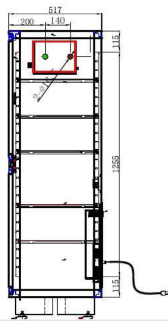
Seitenansicht
